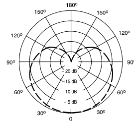
극성 패턴
