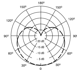
Typische Richtcharakteristik
