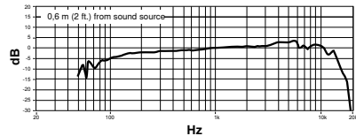
Typischer Frequenzgang
