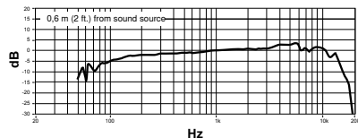
Respuesta de frecuencia típica
